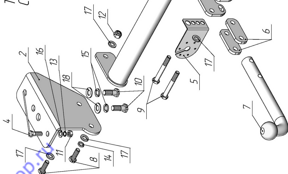
ТСУ "H301-A" Схема сборки
